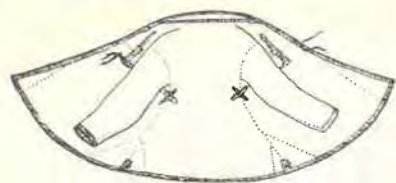
① MORSIESTURKKI KIRVU --- A 6260
